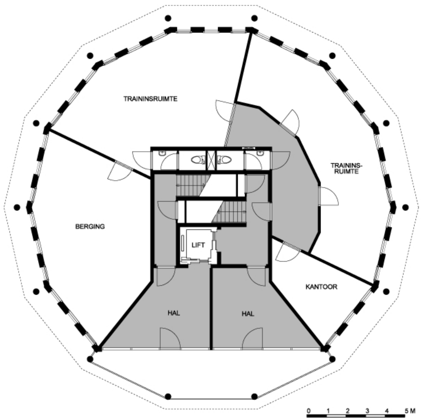
BEGANE GROND
