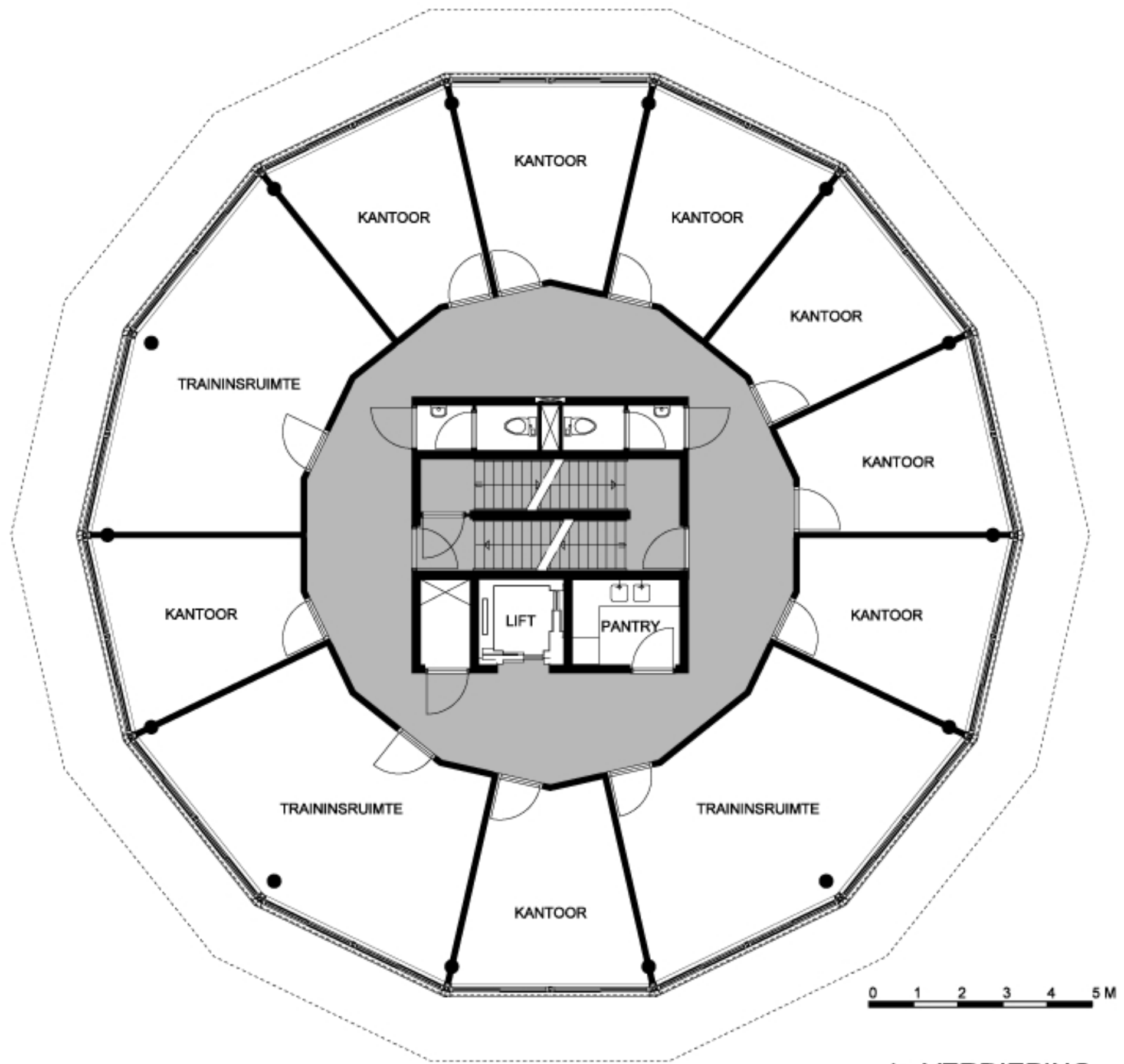
1e VERDIEPING
